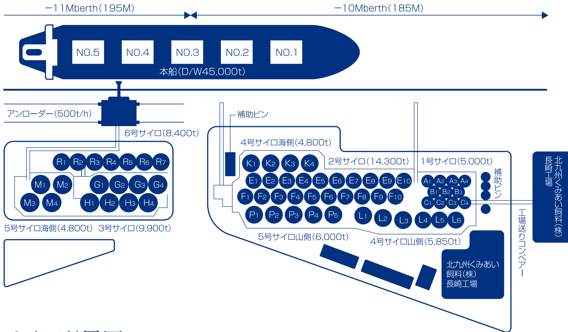
サイロ配置図
